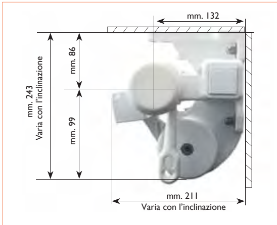
Attacco parete/soffitto
