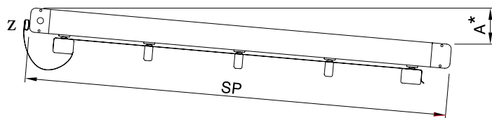
Dimension toile repliée et inclinaison min. avec toile tendue
